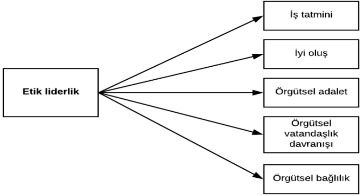
Şekil 1. Etik liderliğin sonuçlarına ilişkin kuramsal model önerisi
