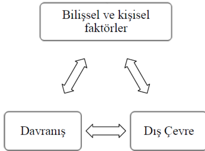
Şekil 1. Davranış, bilişsel ve kişisel faktörler ile dış çevre arasındaki karşılıklı ilişkiler
